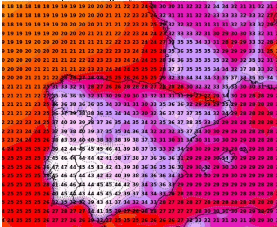
Modellierte Höchsttemperatur für Samstag, 4. August 2018 nach dem amerikanischen GFS-Modell
